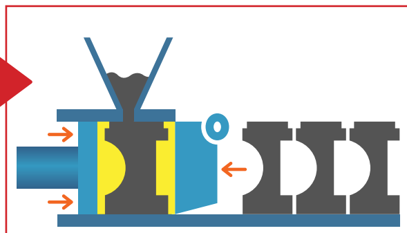
2. Compactação de areia e conformação do molde
