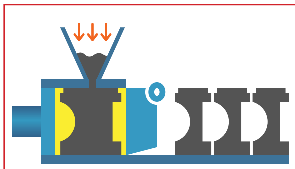
1. Injeção de areia na câmara de moldagem
